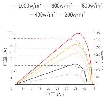
电流 - 电压 & 功率 - 电压曲线图 (480W)
