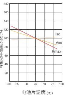
I sc , V oc , P max 的温度曲线
