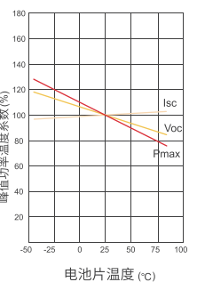
I sc , V oc , P max 的温度曲线
