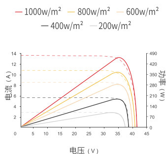
电流 - 电压 & 功率 - 电压曲线图 (460W)
