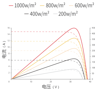
电流 - 电压 & 功率 - 电压曲线图 (450W)
